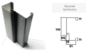
Ościeżnica "11" Protect
