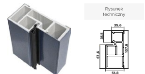
Ościeżnica aluminiowo-kompozytowa Premium
