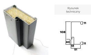
Ościeżnica "11" Protect
