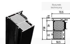
Ościeżnica Alu Hybrid
