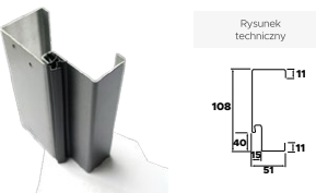
Przekrój drzwi ALU Fireline
