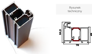
Ościeżnica aluminiowo-kompozytowa Premium
