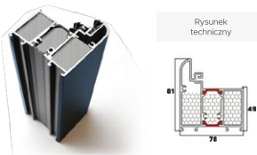
Ościeżnica aluminiowo-kompozytowa Optimum
